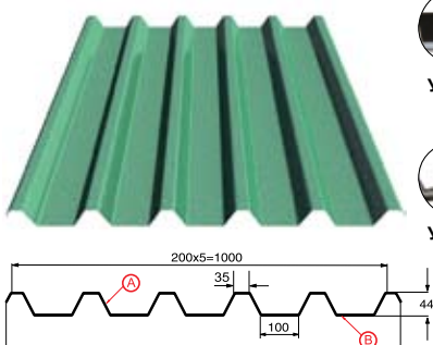
Профилированный лист С-44х1000-А,В Толщина металла 0.5 - 0.8 мм
