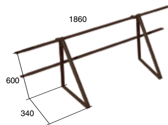
Ограждения кровельные ОК- h600x1860 и ОК- h1200x1860
