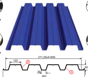
Профилированный лист Н-60х845-А,В Толщина металла 0.5 - 1.0 мм
