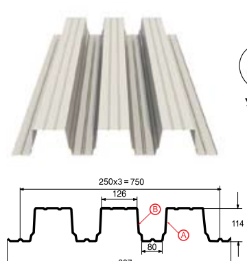
Профилированный лист Н-114х750-А,В Толщина металла 0.8 - 1.0 мм
