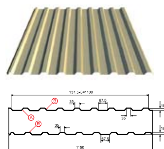
Профилированный лист МП-20х1100-А,В,Р Толщина металла 0.4 - 0.8 мм
