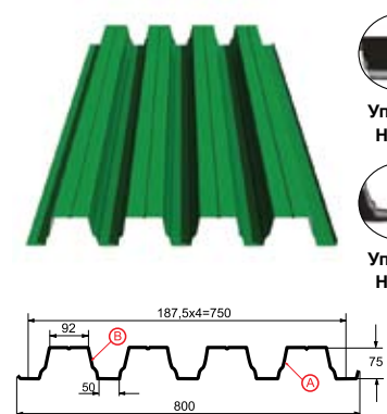
Профилированный лист Н-75х750-А,В Толщина металла 0.7 - 1.0 мм
