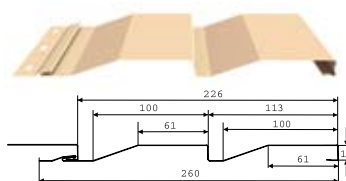
Стальной сайдинг МП СК-14x226
