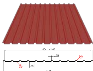
Профилированный лист С-10х1100-А,В Толщина металла 0.4 - 0.7 мм Производится в СФО
