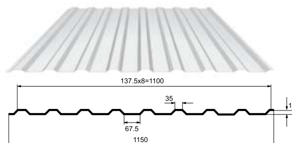
Поликарбонатный профилированный лист МП-20x1100 Толщина поликарбоната 0.9 мм
