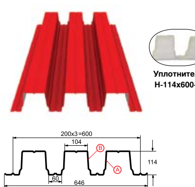
Профилированный лист Н-114х600-А,В Толщина металла 0.8 - 1.0 мм
