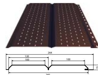
Софит Лбрус (перфорированный) для подшивки карнизных свесов
