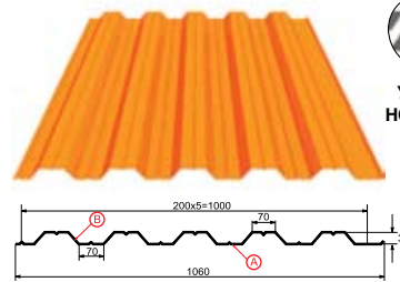
Профилированный лист НС-35х1000-А,В Толщина металла 0.5 - 0.9 мм
