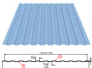
Профилированный лист С-8х1150-А,В Толщина металла 0.4 - 0.7 мм
