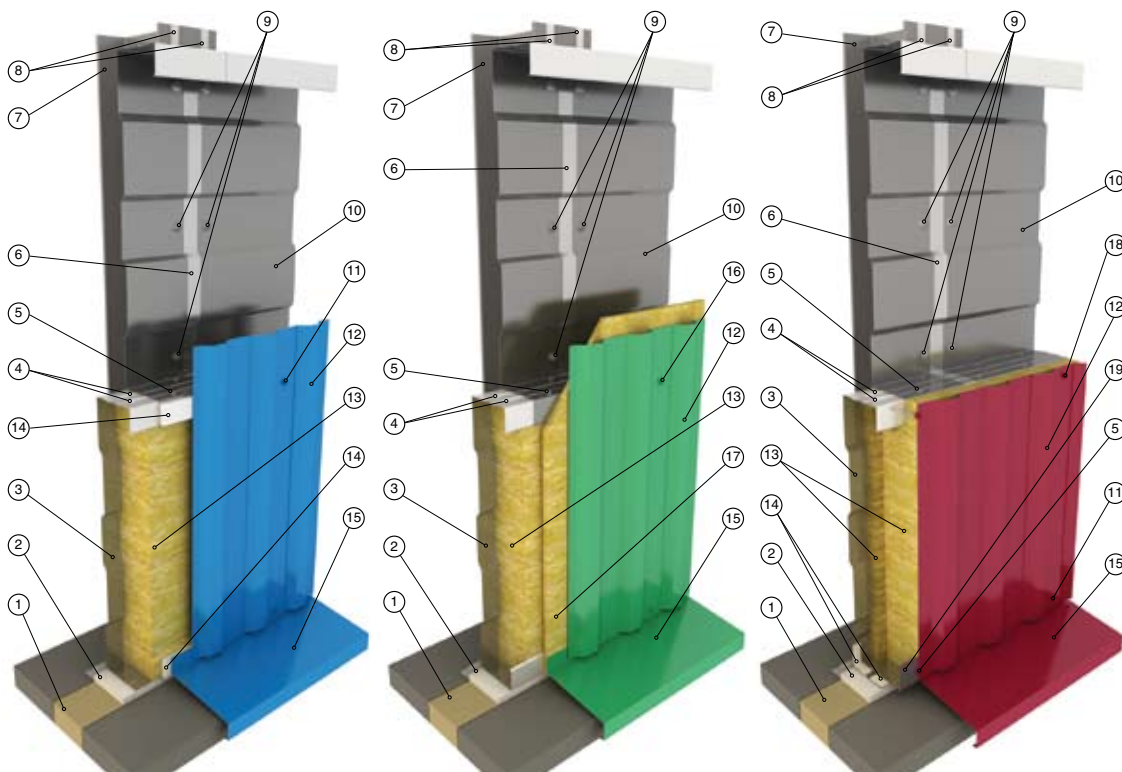
Варианты Юг-100 (вар.ТП или МВ) или 150 (вар.ТП или МВ). Общая толщина теплоизоляции 100 или 150 мм.
