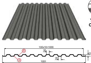
Профилированный лист С-21х1000-А,В Толщина металла 0.4 - 0.7 мм
